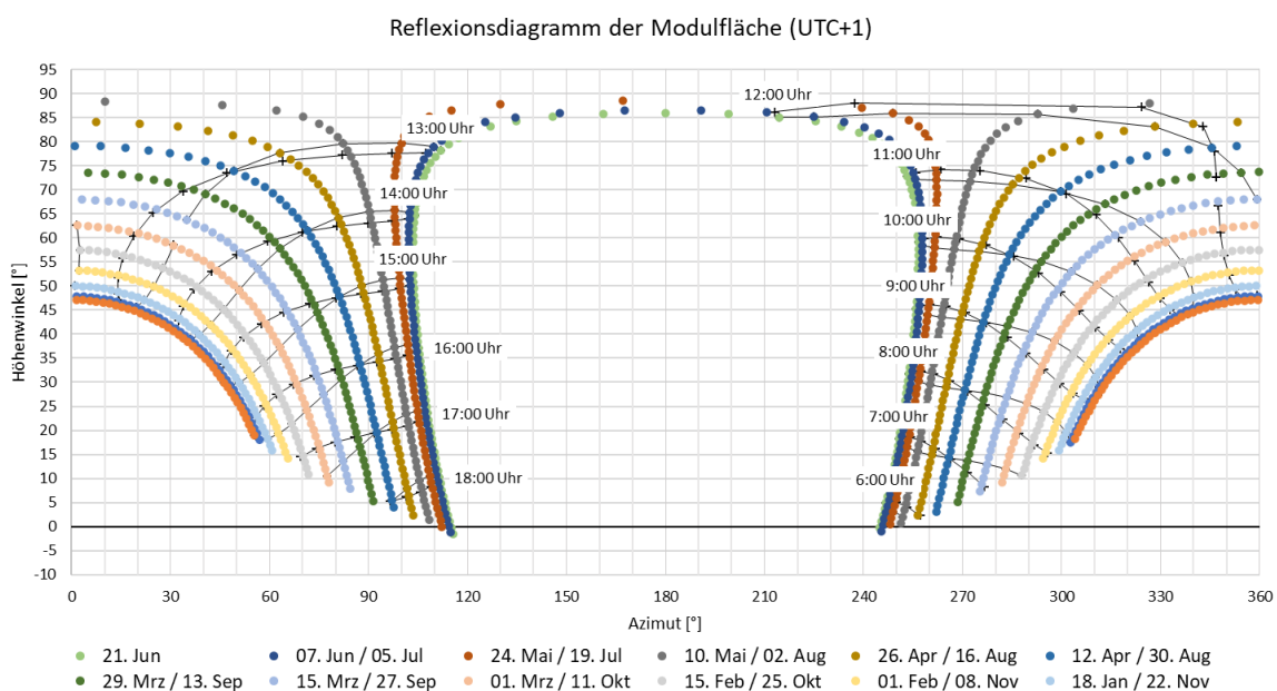
Abbildung 11: Reflexionsdiagramm für den Standort Niedermurach Sallach mit einem Azimutwinkel von 180^\circ und einem Modulneigungswinkel von 15^\circ
