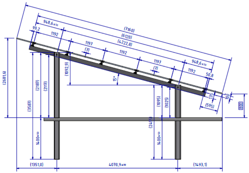
Abbildung 3: Maße der Unterkonstruktion (Quelle: Auftraggeber)
