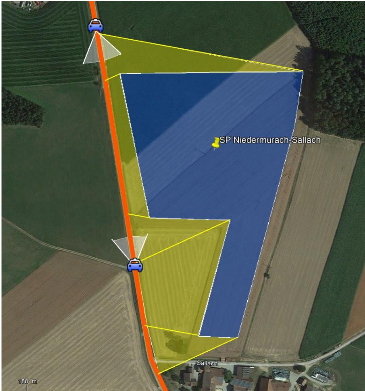
Abbildung 12: Emissionswinkel der PV-Fläche und Immissionswinkel der Straßenverkehrsteilnehmer mit Blickwinkelberücksichtigung von \pm 30^\circ
